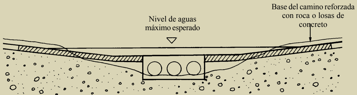
b. Vado simple mejorado o con tubos de alcantarillas en un cauce ancho.
