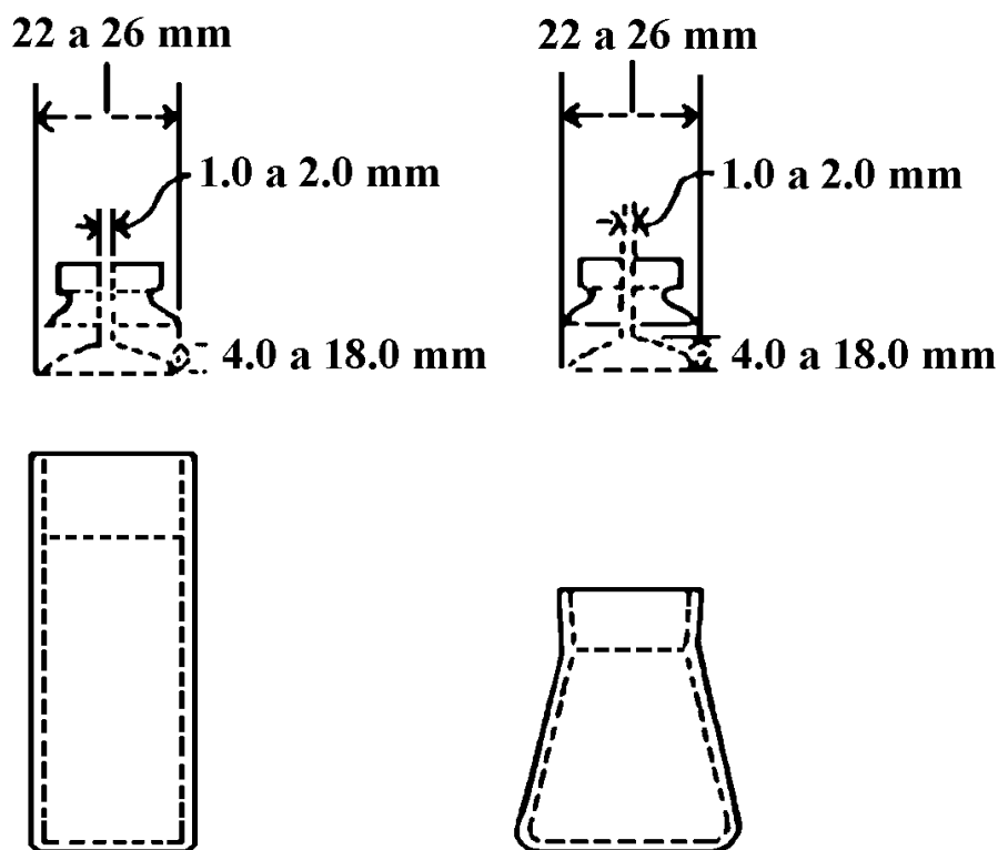
FIGURA 9. Pícnómetros
