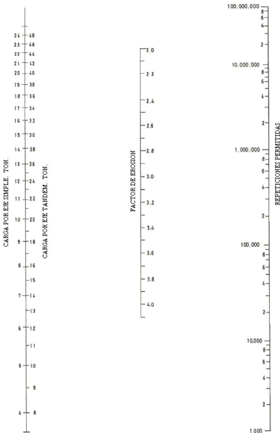
Figura IX.3. Método PCA 1984, análisis por erosión - acotamiento sin pavimento. Fuente: Guía para el Diseño y la Construcción de Pavimentos Rígidos. Ing. Aurelio Salazar Rodríguez, 1998.
