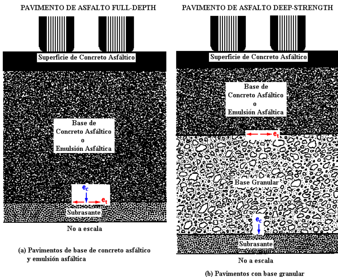
Figura VI.3. Localización de los esfuerzos considerados en el procedimiento de diseño. Fuente: Asphalt Institute's Thickness Design Manual (MS-1)
