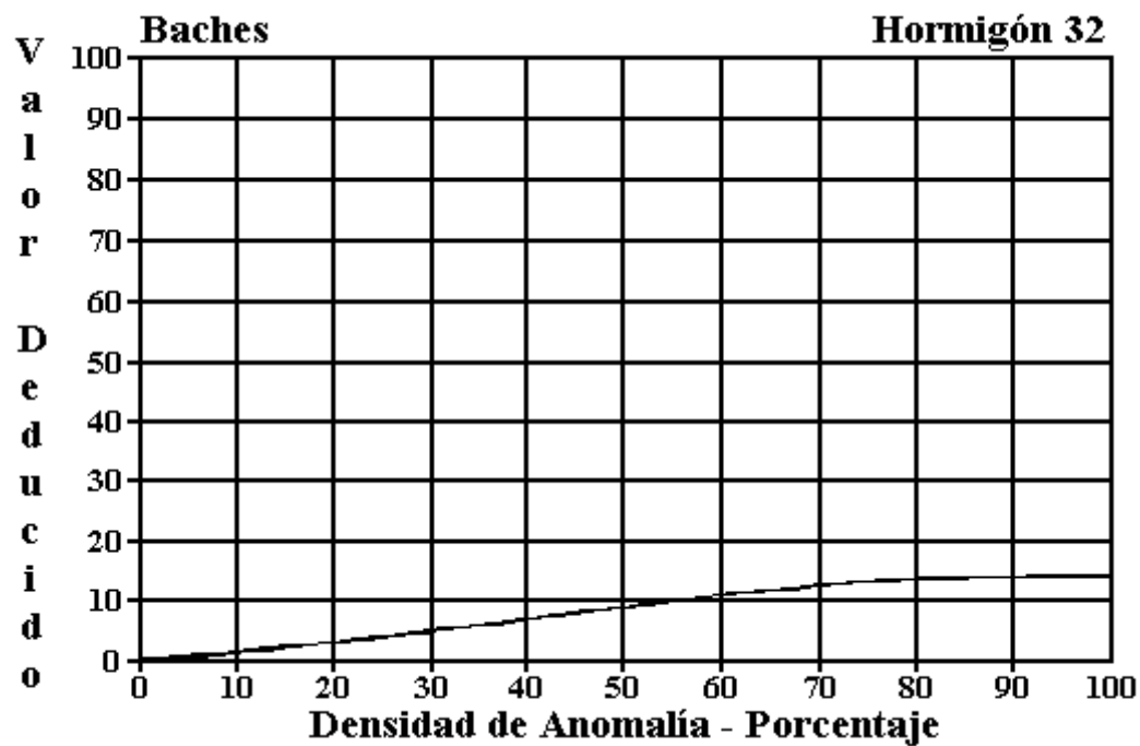
Figura C-31. Baches.
