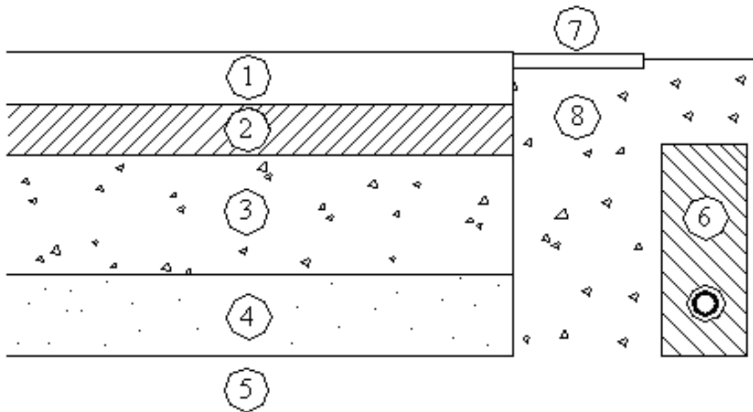
Figura I.1. Sección típica de un pavimento.
