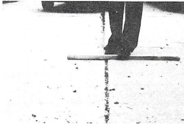
Figura C-5.a. Falla Baja-severidad.
