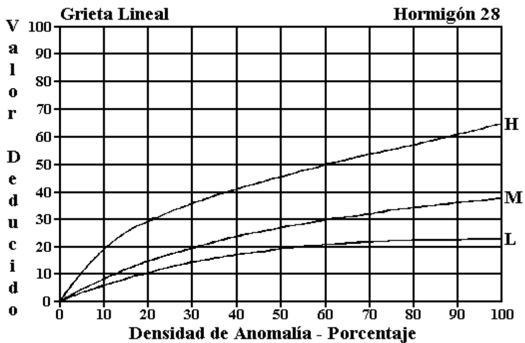
Figura C-27. Agrietamiento Lineal.
