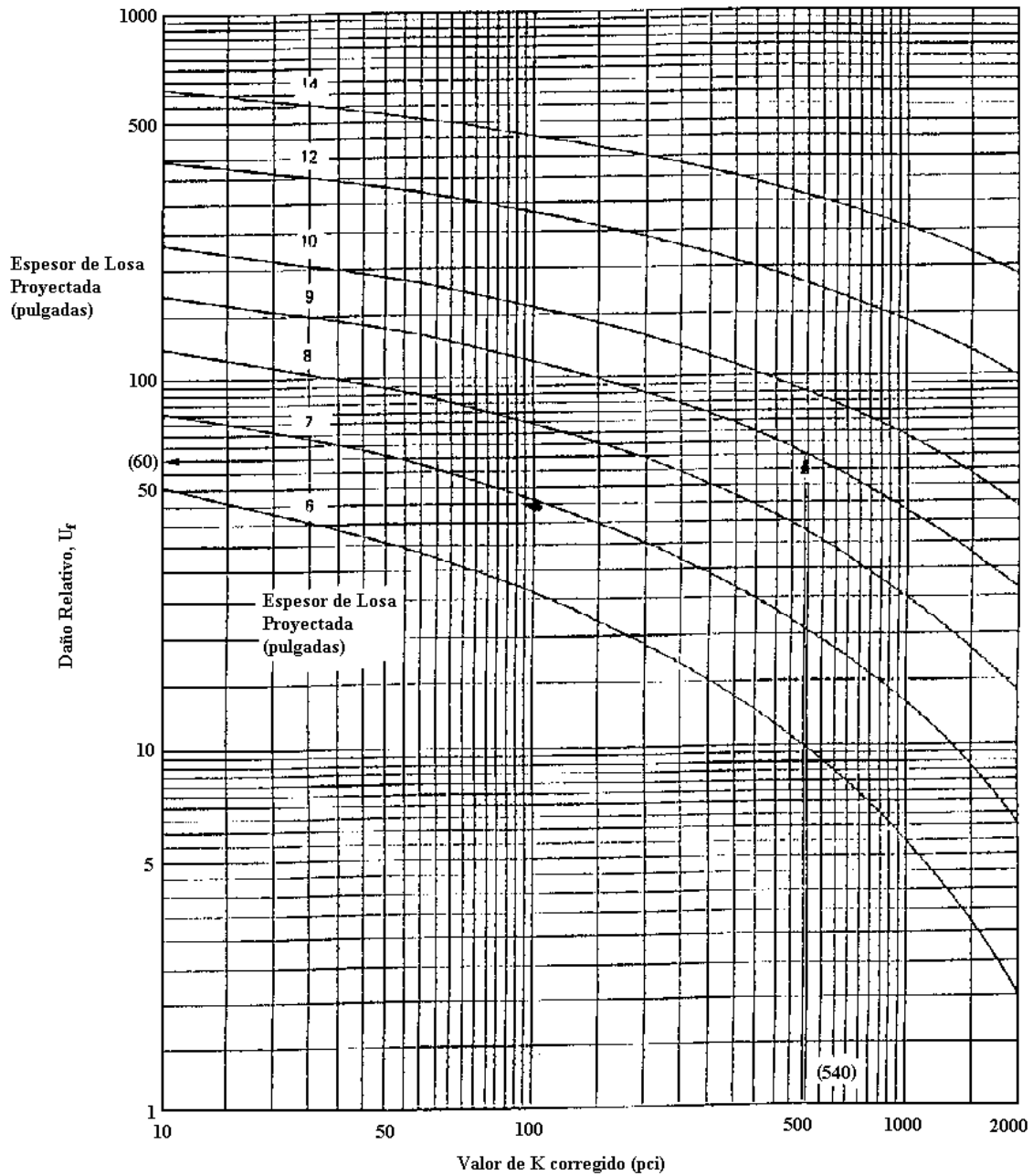
Figura. VIII.2. Daño Relativo del Pavimento Rígido. Fuente: Guide for Design of Pavement Structures, AASHTO, 1993.
