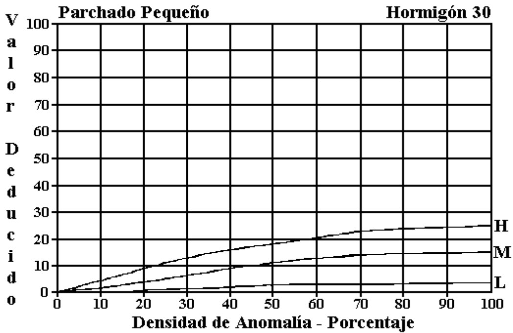
Figura C-29. Parchado Pequeño.
