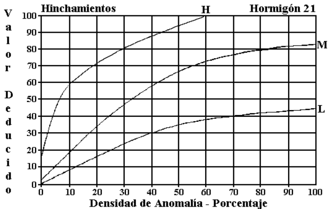
Figura C-20. Hinchamiento / Pandeo.
