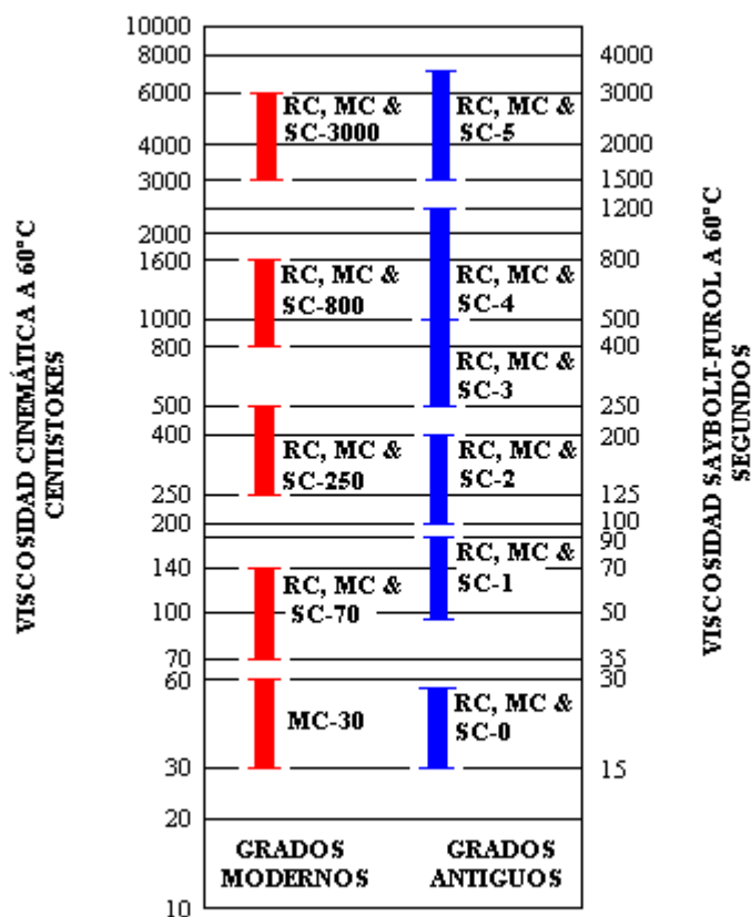
Figura II.2. Comparación de los grados antiguos y modernos de asfalto líquido. Fuente: The Asphalt Institute's, Manual del Asfalto.
