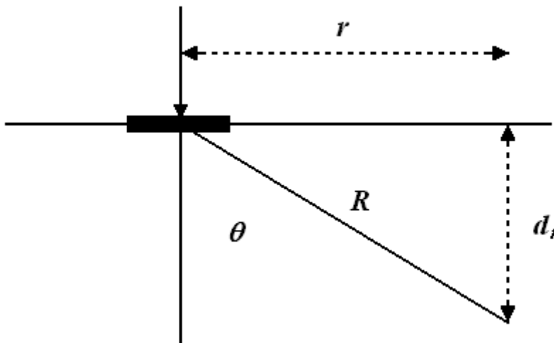
Figura XI.2. Distancia a la que la deflexión depende sólo de las propiedades de la subrasante.
