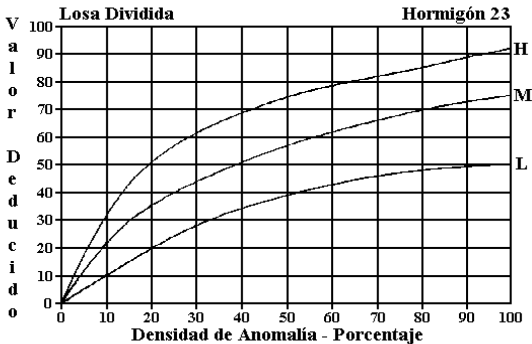
Figura C-22. Losa Dividida.
