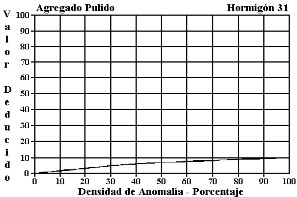
Figura C-30. Agregado Pulido.
