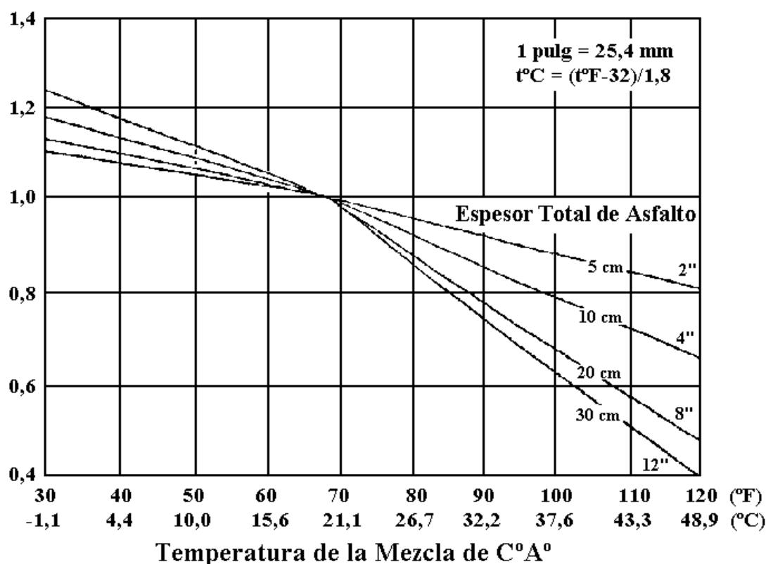
Figura XI.5. Ajuste para d_0 por temperatura para pavimento con base tratada con cemento y/o puzolanas.
