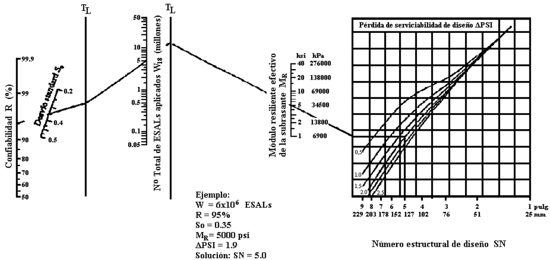
Figura IV.2. Ábaco de diseño AASHTO para pavimentos flexibles. Fuente: AASHTO, Guide for Design of Pavement Structures 1993
