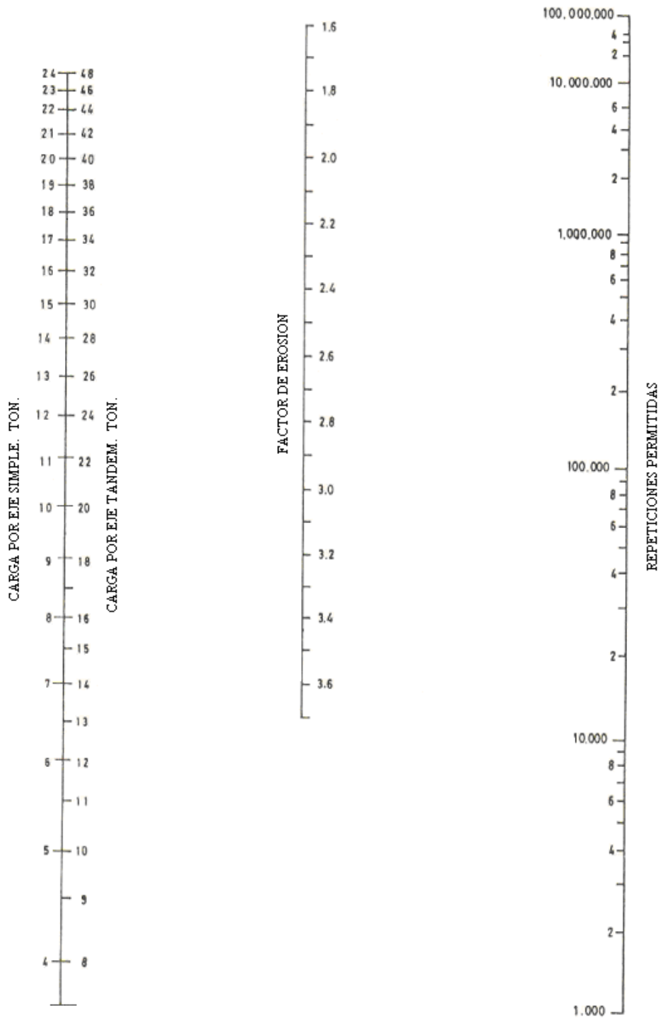
Figura IX.4. Método PCA 1984, análisis por erosión - acotamiento pavimentado. Fuente: Guía para el Diseño y la Construcción de Pavimentos Rígidos. Ing. Aurelio Salazar Rodríguez, 1998.
